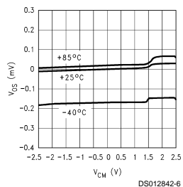
V_{OS} vs V_{CM} V_S = \pm 2.5\text{V}
