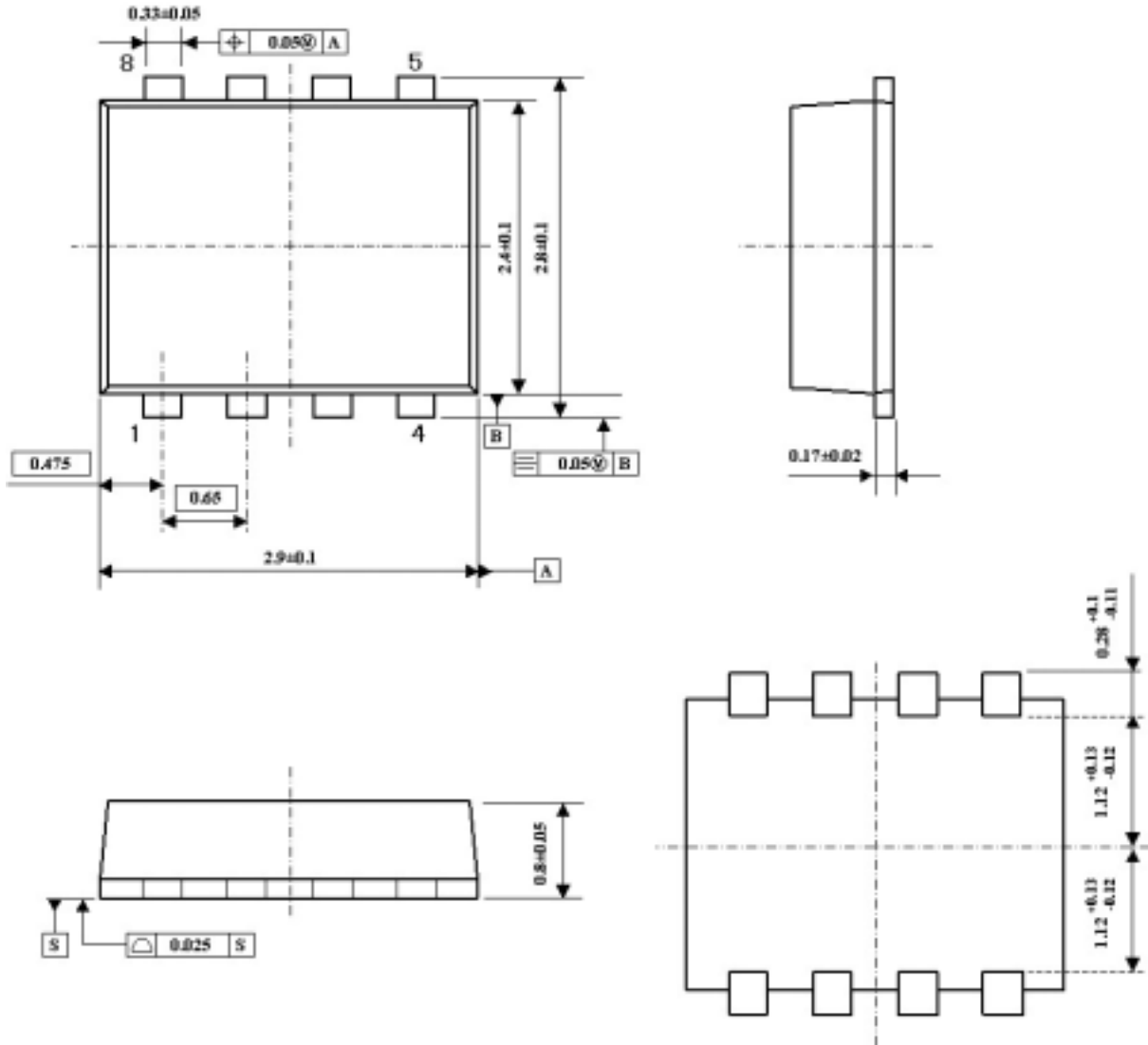
注 7: 外形图
