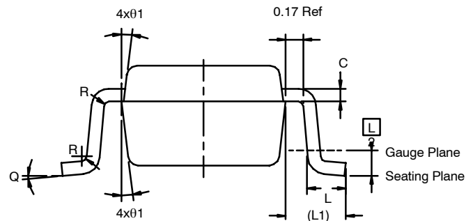
SOT23-6L Format
