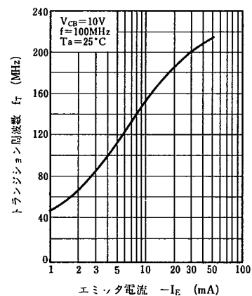
f_T - I_E
