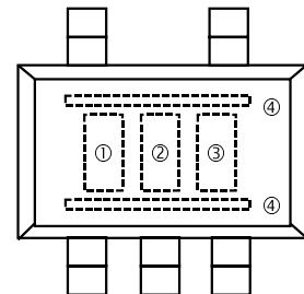
(3) SOT-23-5
