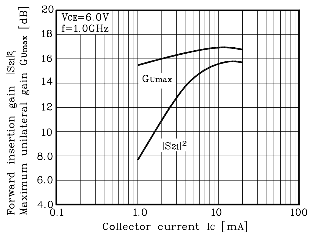
Fig. 11 |S 21 | 2 ,G Umax -I C
